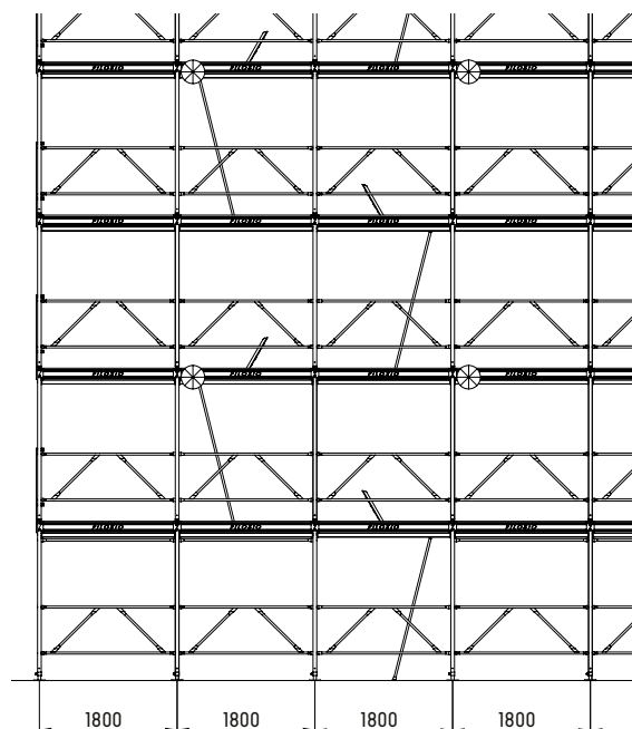
Schema K105 con telaio parapetto doppio.
