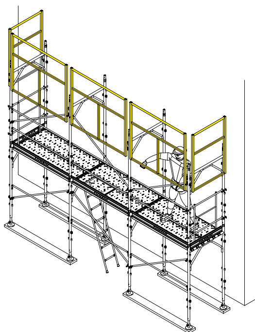
Montaggio del ponteggio IN SICUREZZA con parapetto. Utilizzabile con ponteggi K, KZ e PE.
