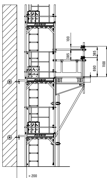
Piazzola di carico.
