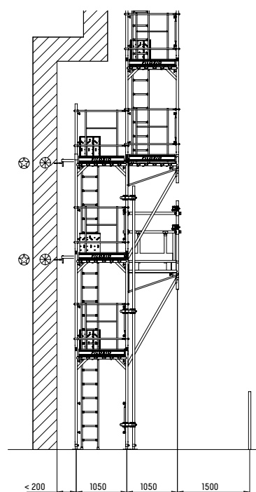
Mensola per sbalzo.
