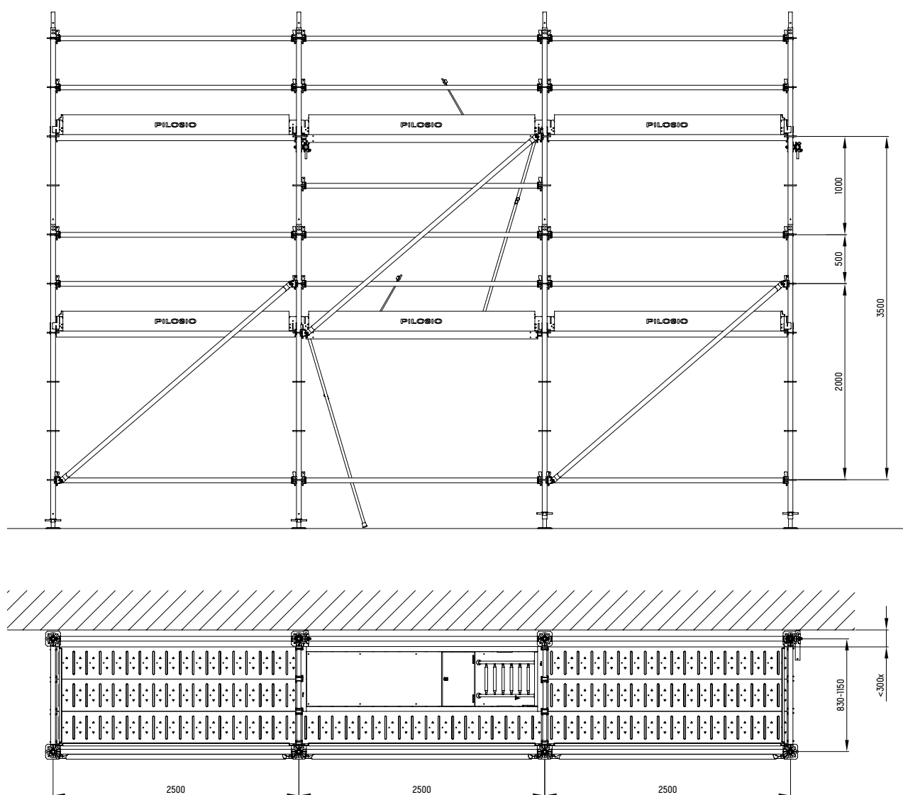
Schema ponteggio multidirezionale MP 83/115 passo 250 cm.
