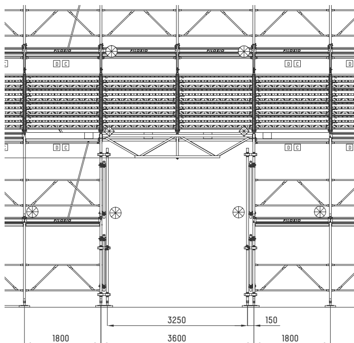
Schema passo carraio KZ105 da 360.
