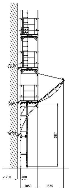
Partenza stretta K e KZ.
