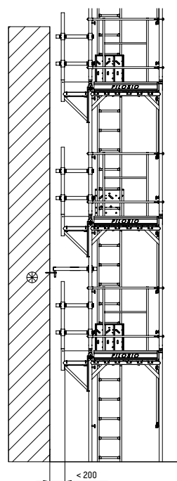
Mensola per piano di lavoro K e KZ.
