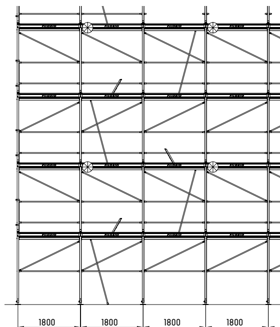
Schema KZ105 con correnti e diagonali.
