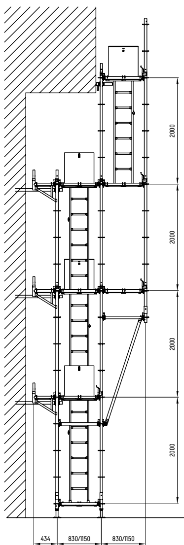
Mensola a sbalzo interna ed esterna.
